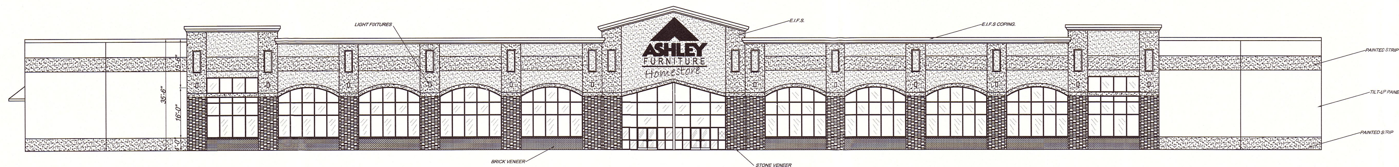
1 FRONT ELEVATION A3 SCALE: 1/16"=1'-0"
